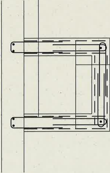
COUPE HORIZONTALE
